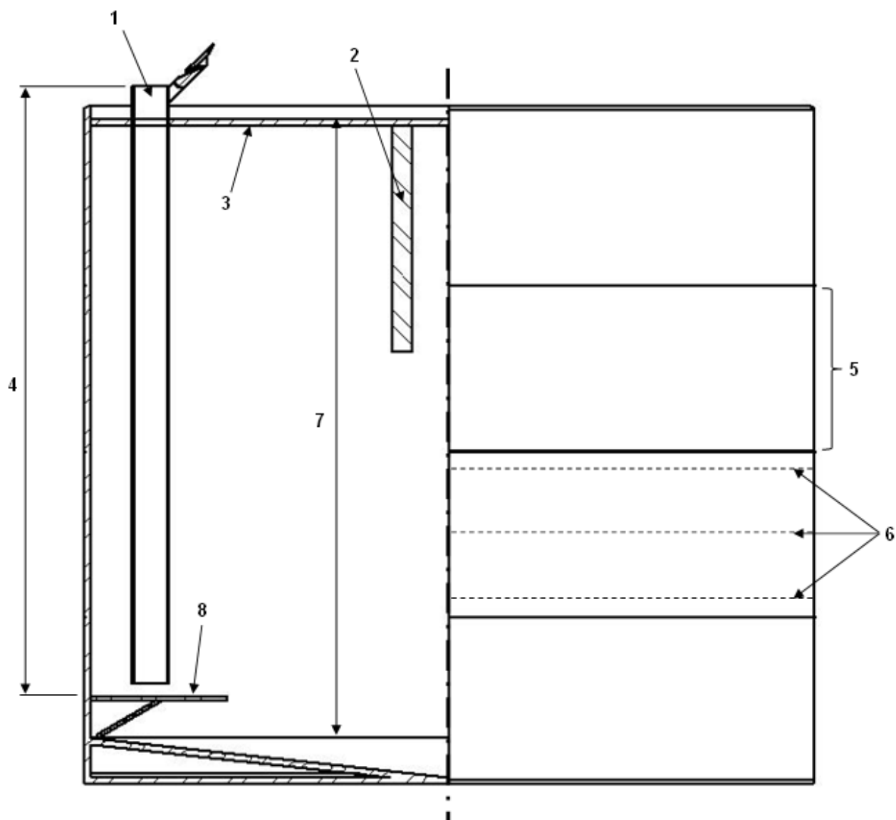
Figura 1 – Desenho esquemático de tanque cilíndrico vertical.
