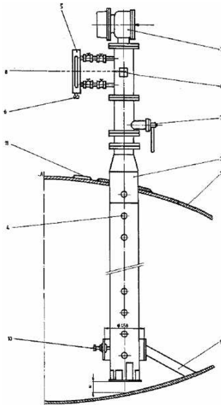
Figura 9 – Desenho esquemático de um tanque esférico pressurizado.
